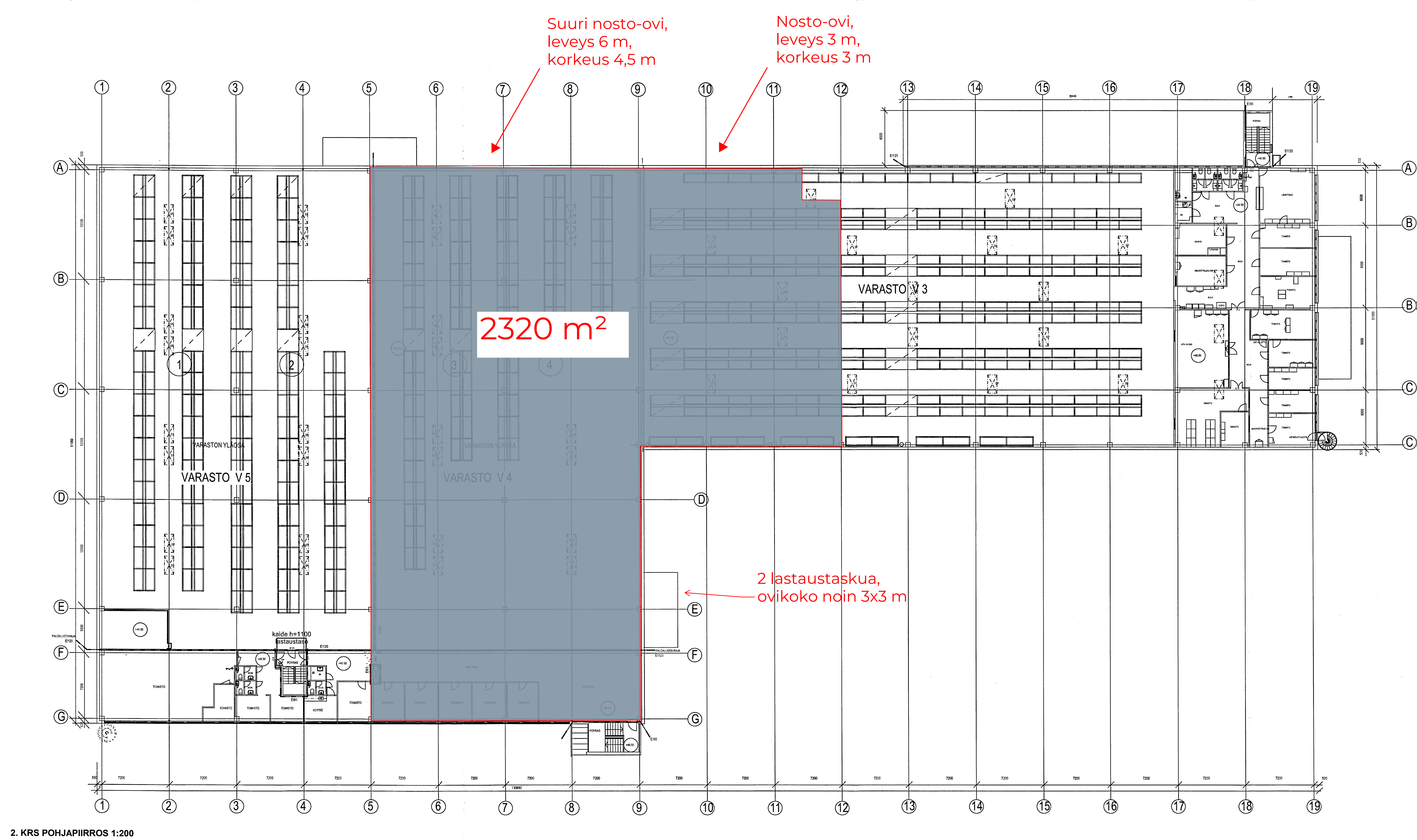
2. KRS POHJAPIIRROS 1:200
