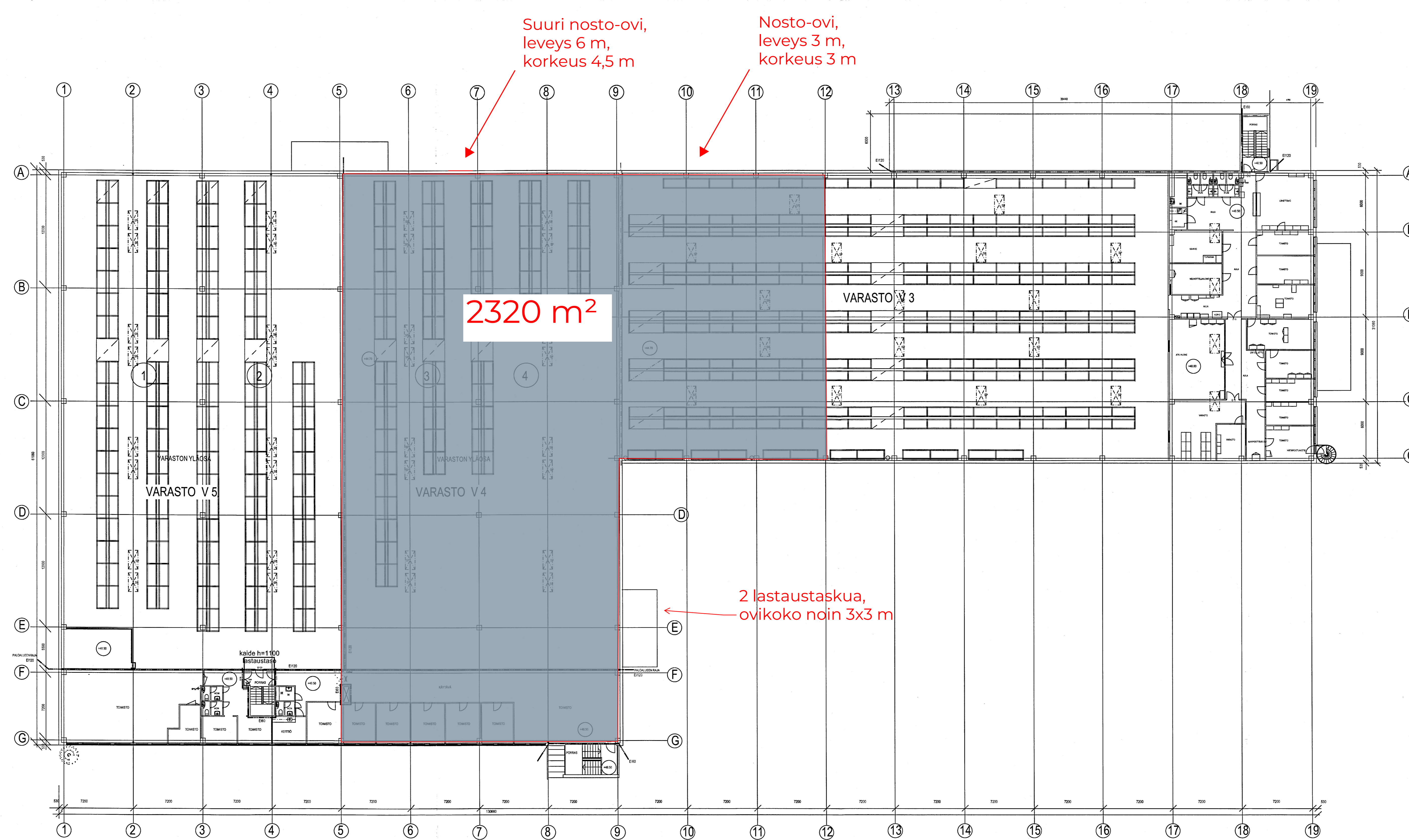
2. KRS POHJAPIIRROS 1:200
