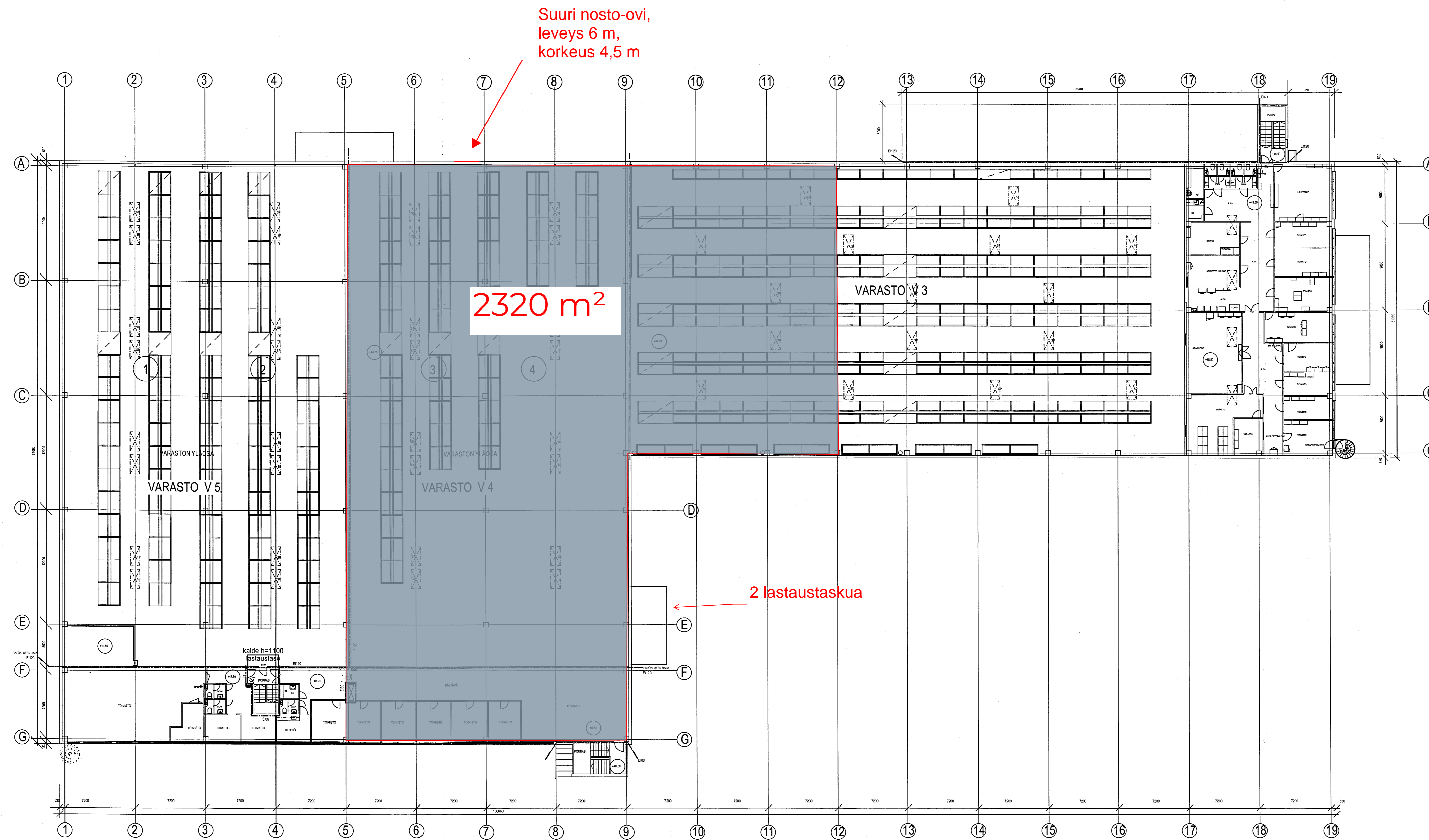
2. KRS POHJAPIIRROS 1:200
